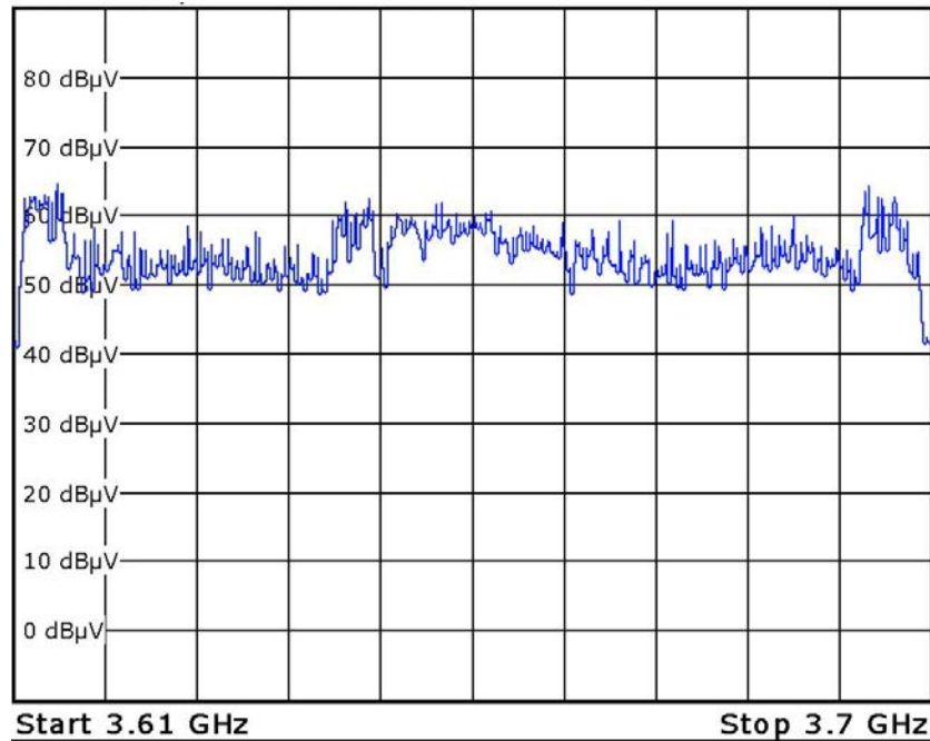
Abb. 12: Die Kanalbandbreite von 90 MHz kann vom Signal maximal zu 95 % ausgeschöpft werden (85,5 MHz), wie es hier der Fall ist
