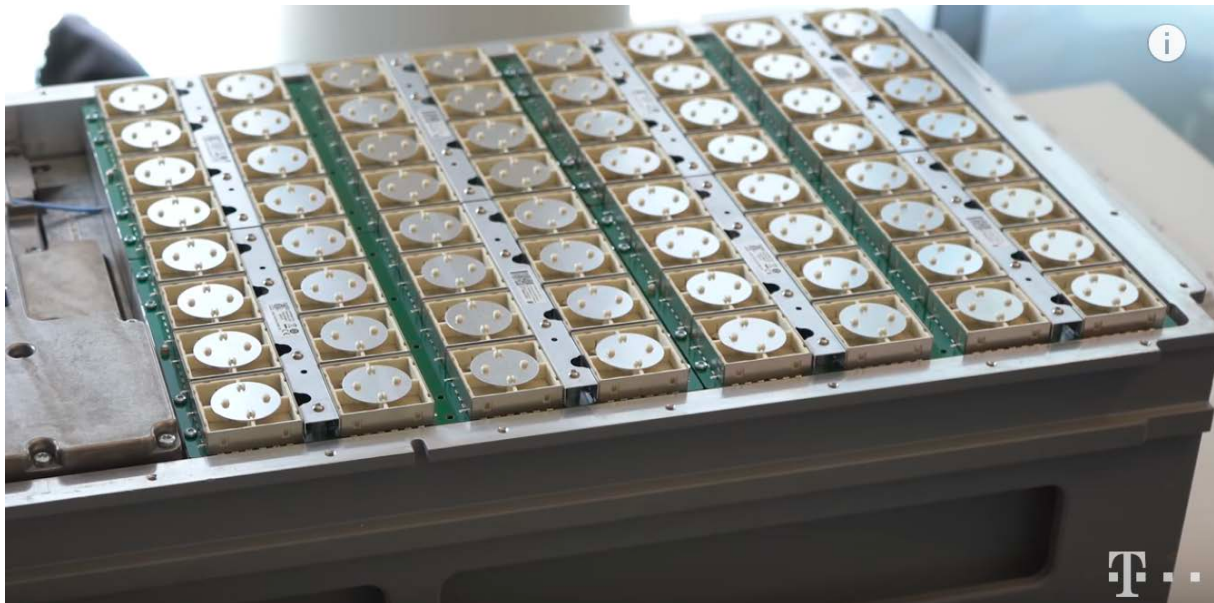
Abb. 11: „Smarte Antenne“ mit aktivem Beamforming, Gehäusedeckel entfernt, so dass das 8 x 8 Array mit 64-MIMO sichtbar ist [23]; Antenne gegenüber Abb. 10 um 90° gedreht.
