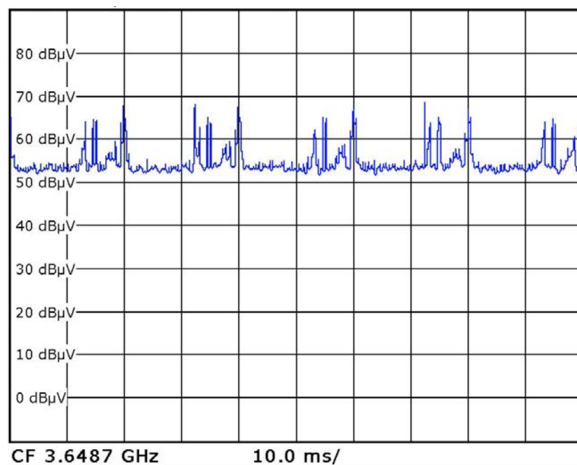
Abb. 16: Zeitverlauf des 5G NR-Signals bei gröberer zeitlicher Auflösung: Zeitskala 100 ms bzw. 10 ms pro Teilung.
