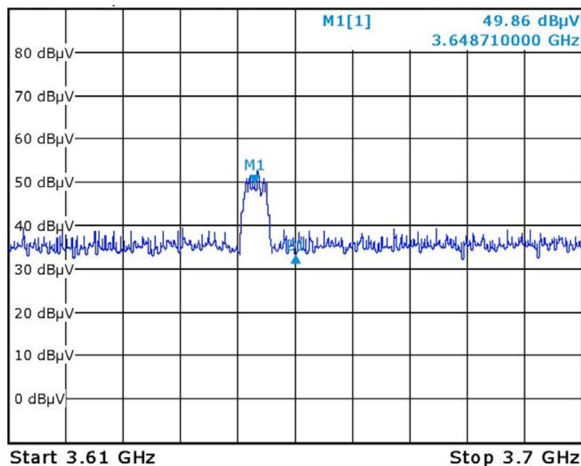
Abb. 14: Hier sind nur die permanent im 50Hz-Rhythmus ausgesendeten, verkehrslastunabhängigen Synchronisierungs-Signale ( Primary Synchronization Signal PSS und Secondary Synchronization Signal SSS ) sowie der Physical Broadcast Channel PBCH aktiv, die gemeinsam im SSB ( Synchronization Signal Block ) gesendet werden und die Grundlast ausmachen, wenn über die Basisstation keine Verkehrslast (Traffic) läuft und die Anlage sich sozusagen im Leerlauf befindet.
