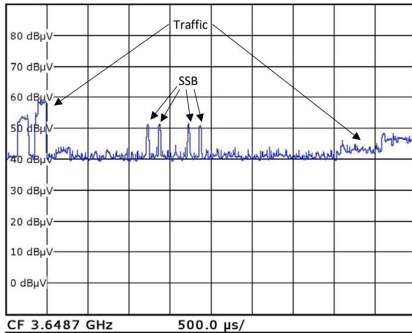
Abb. 15: Zeitverlauf des 5G NR-Signals bei Abstimmung des Analysators auf die Mitte des SSB (Center Frequenz CF 3,6487 GHz, vgl. Abb. 14), mit Zeitskala 5 ms bzw. 500 µs pro Teilung.
