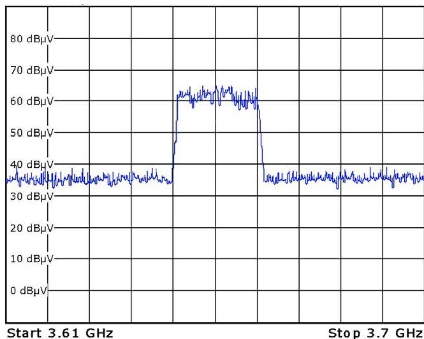
Abb. 13: Zu diesem Zeitpunkt sind nur Endgeräte aktiv, die keine sehr hohen Anforderungen an Übertragungskapazität und Bandbreite haben; die Basisstation passt sich automatisch dem Bandbreitebedarf der Endgeräte an.
