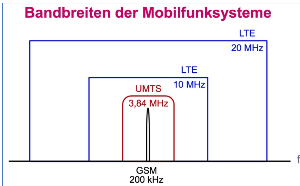
Abb. 2: Bandbreiten der Mobilfunksysteme 2 G bis 4 G
